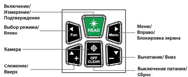
Рис. 4 Кнопки управления
